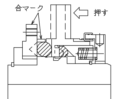
リリース時 (オーバーロード)
