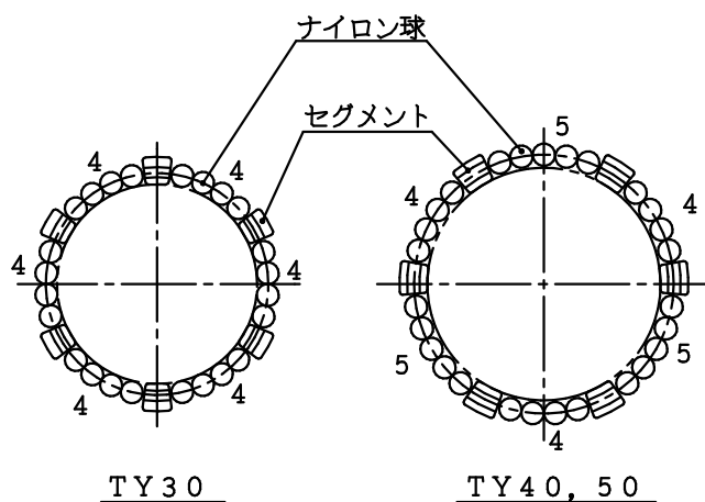
セグメントおよびナイロン球組み配置図
